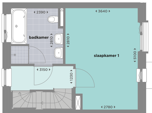
Eerste verdieping
