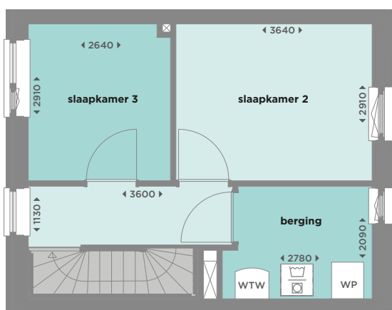
Tweede verdieping
